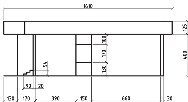
شکل ۹-۲. نقشه نماهای ساختمان
